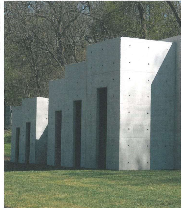
Fotomeenus mullusest võitjast: Tallinna lauluväljakul asuv heliskulptuur Cromatico. Idee autor skulptor Lukas Kühne; konstruktor – Andrei Kervališvili, Nordecon Betoon OÜ; ehitaja Nordecon Betoon OÜ; betooni tarnija – HC Betoon AS.
